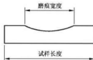
图 1 磨痕宽度
