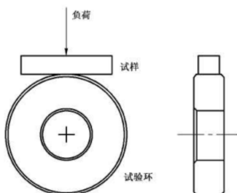
图2 试验示意图
